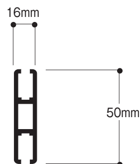
ビーム断面図
